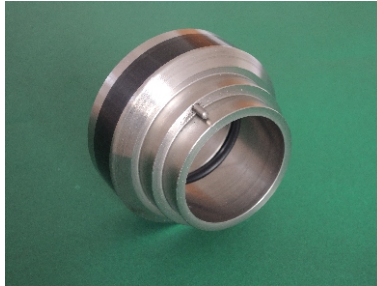
Tulejka uszczelnienia BWLKH 33mm 1,4571 wersja płukana
