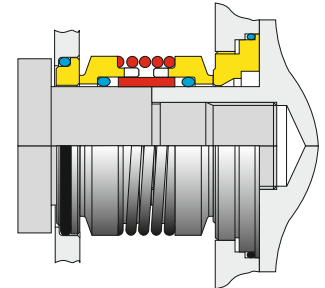
Uszczelnienie podwójne
