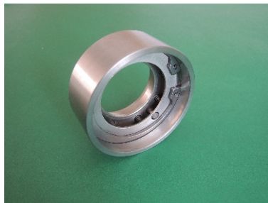
Korpus uszczelnienia BWLKH 32mm 1,4404
