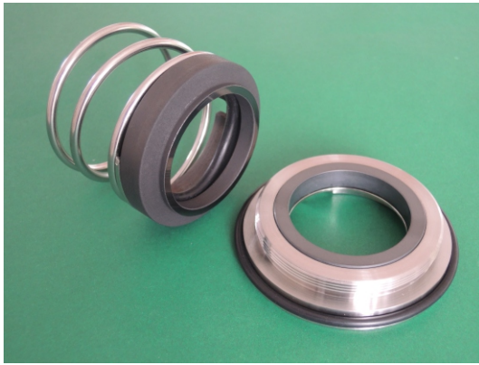
Tulejka uszczelnienia BWLKH 33mm 1,4571 wersja pojedyncza
