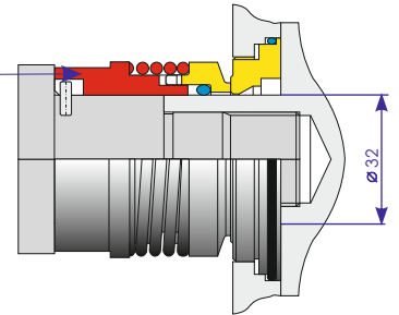
Uszczelnienie pojedyncze
