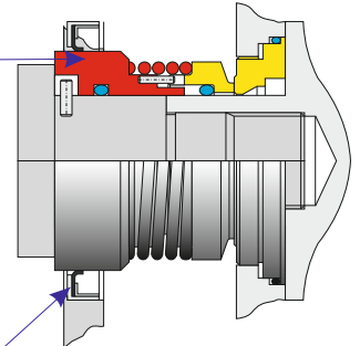
Uszczelnienie płukane
