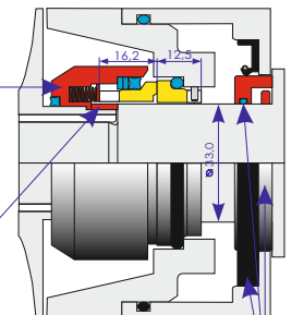
Uszczelnienie płukane
