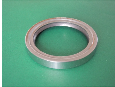
Uszczelka wargowa LIPSEAL BWLKH 33mm wersja płukana
